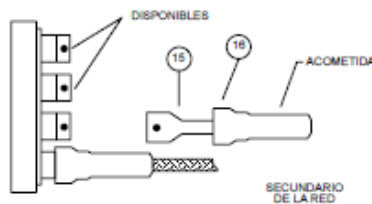
DETALLE "A"
