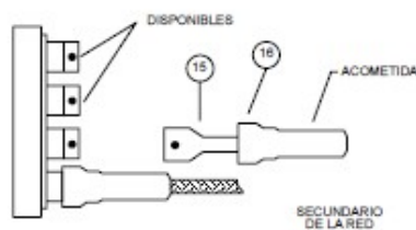
DETALLE "A"
